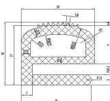
Uszczelka typ e
